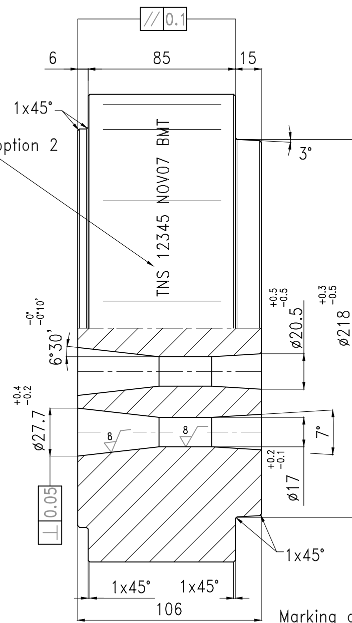
Sec. A-A
